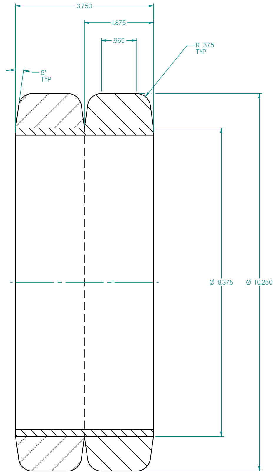
SECTION A-A
